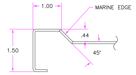
SECTION A-A SCALE: FULL
