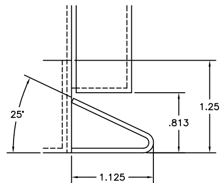
RAMP DETAIL SCALE: 6"=1'-0"
